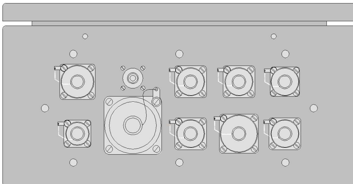
Рис. 3. Прибор ИВЭ-50 модель 201G (разъемы на корпусе)
