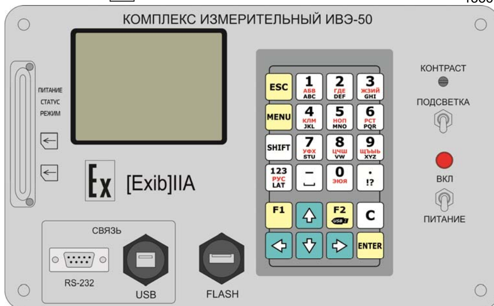
Рис. 1. Прибор ИВЭ-50 модель 101G (крышка с органами управления).
