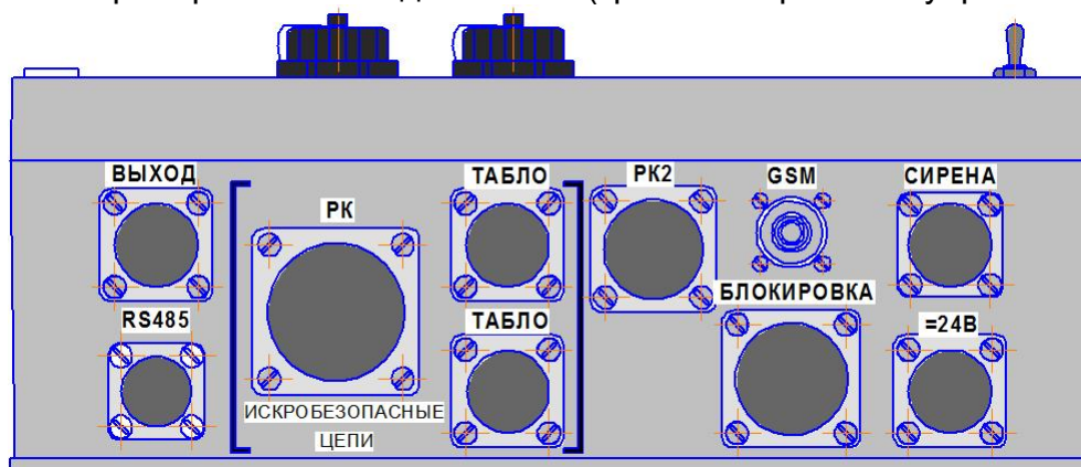
Рис. 1. Прибор ИВЭ-50 модель 101G (крышка с органами управления).
