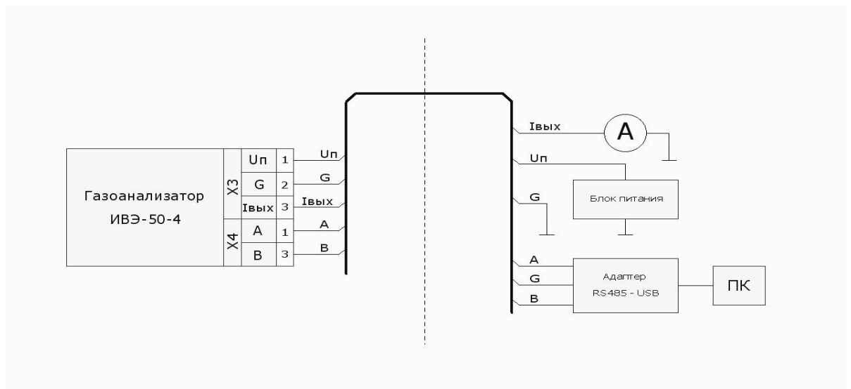
Рис. Б2 - Схема электрических соединений
