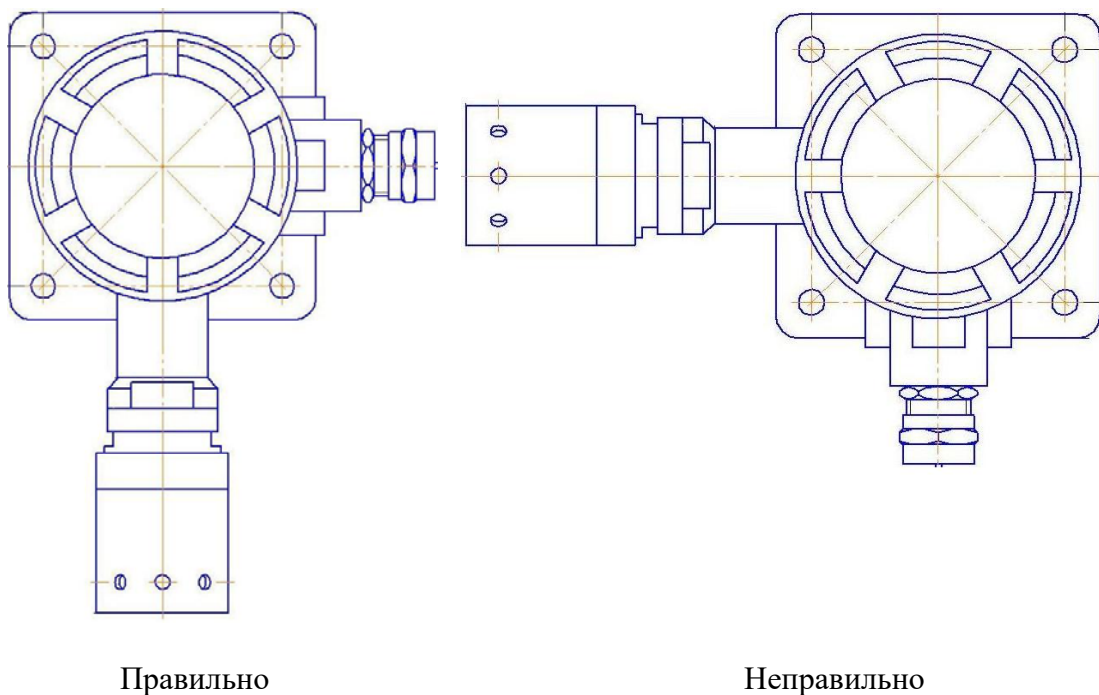
Рис. 4 Способ установки газоанализатора
