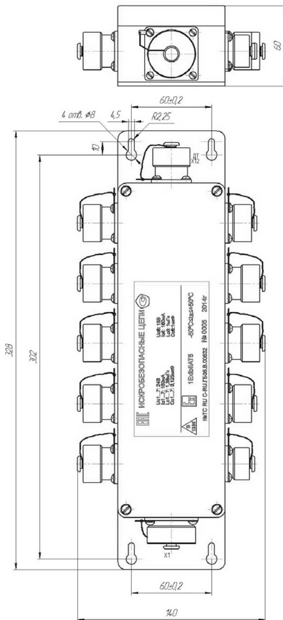
Рис. Коробка распределительная РК32.104. Габаритные размеры.
