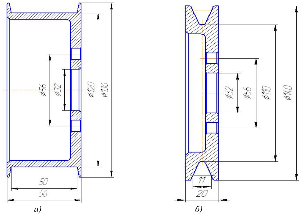
Рис.2. Варианты исполнения шкива с одинаковым креплением к датчику.
