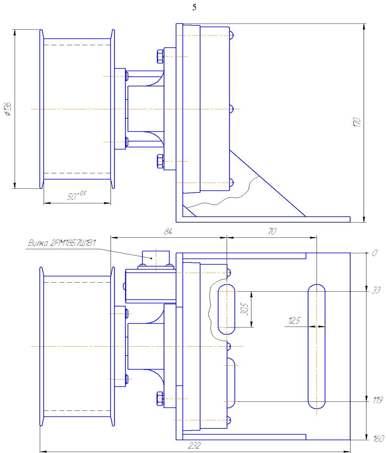
Рис.3 Габаритные и установочные размеры датчика
