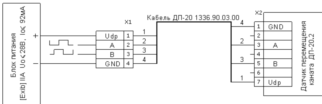
Рис.4 Схема подключения датчика
